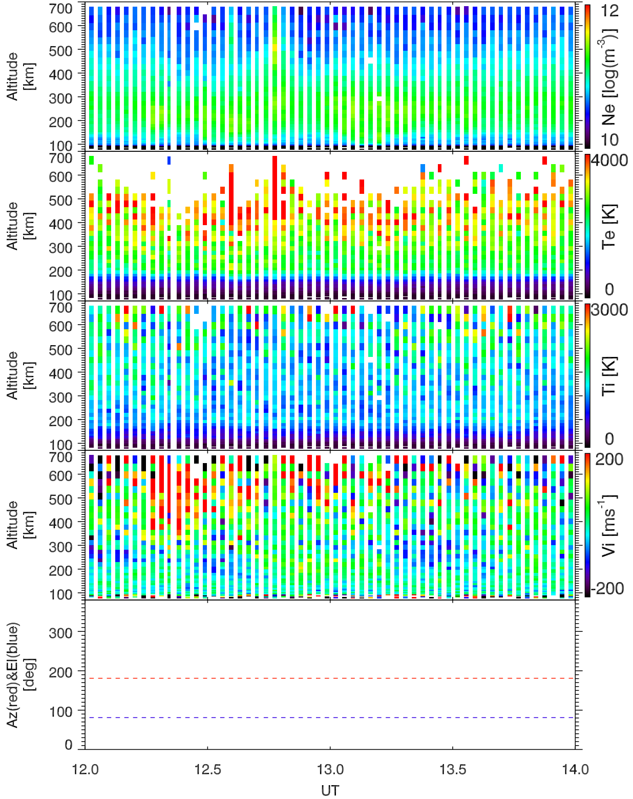
EISCAT 2004-06-09_12_14UT_steffe_ant@42m.
