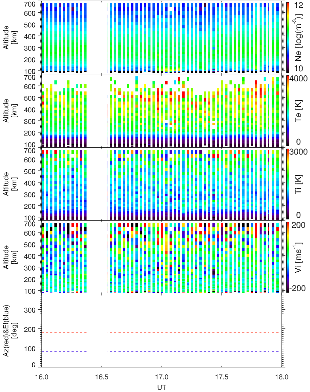
EISCAT 2004-06-09_16_18UT_steffe_ant@42m.
