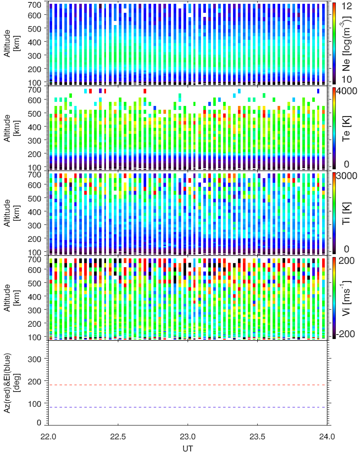
EISCAT 2004-06-09_22_24UT_steffe_ant@42m.
