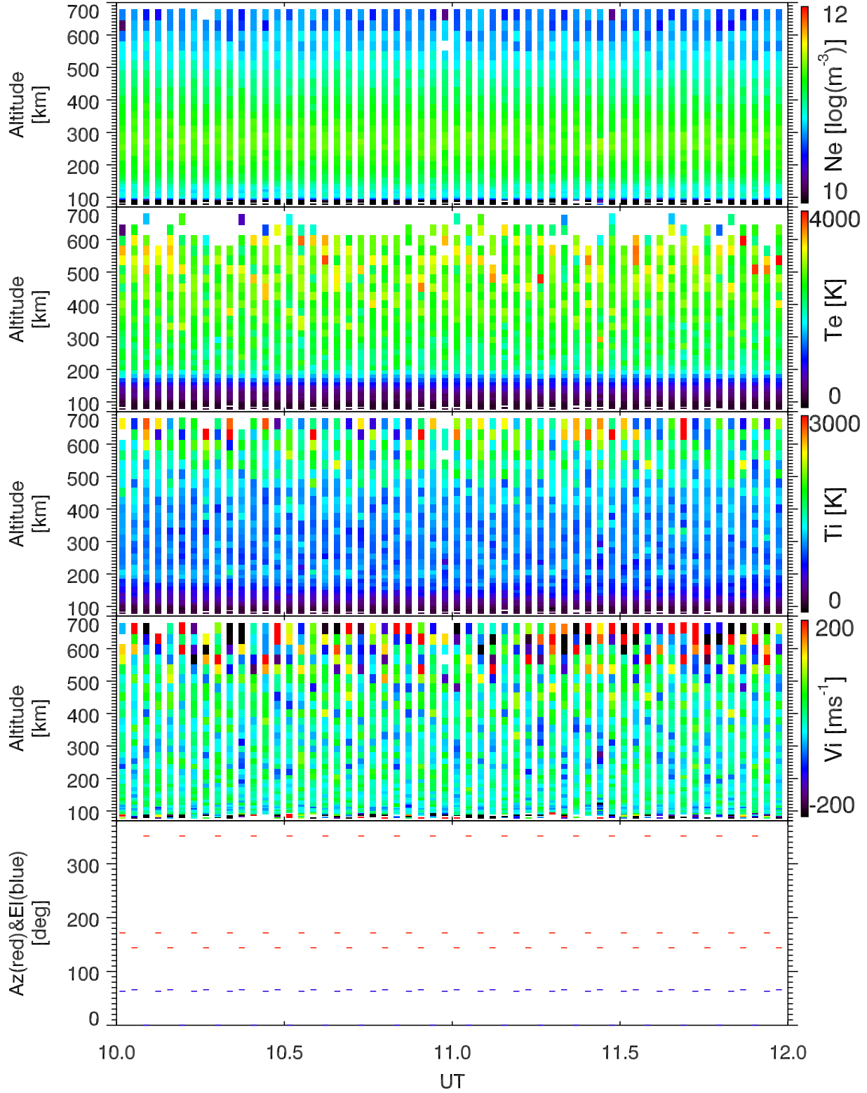
EISCAT 2004-06-10_10_12UT_steffe_ant@32m.
