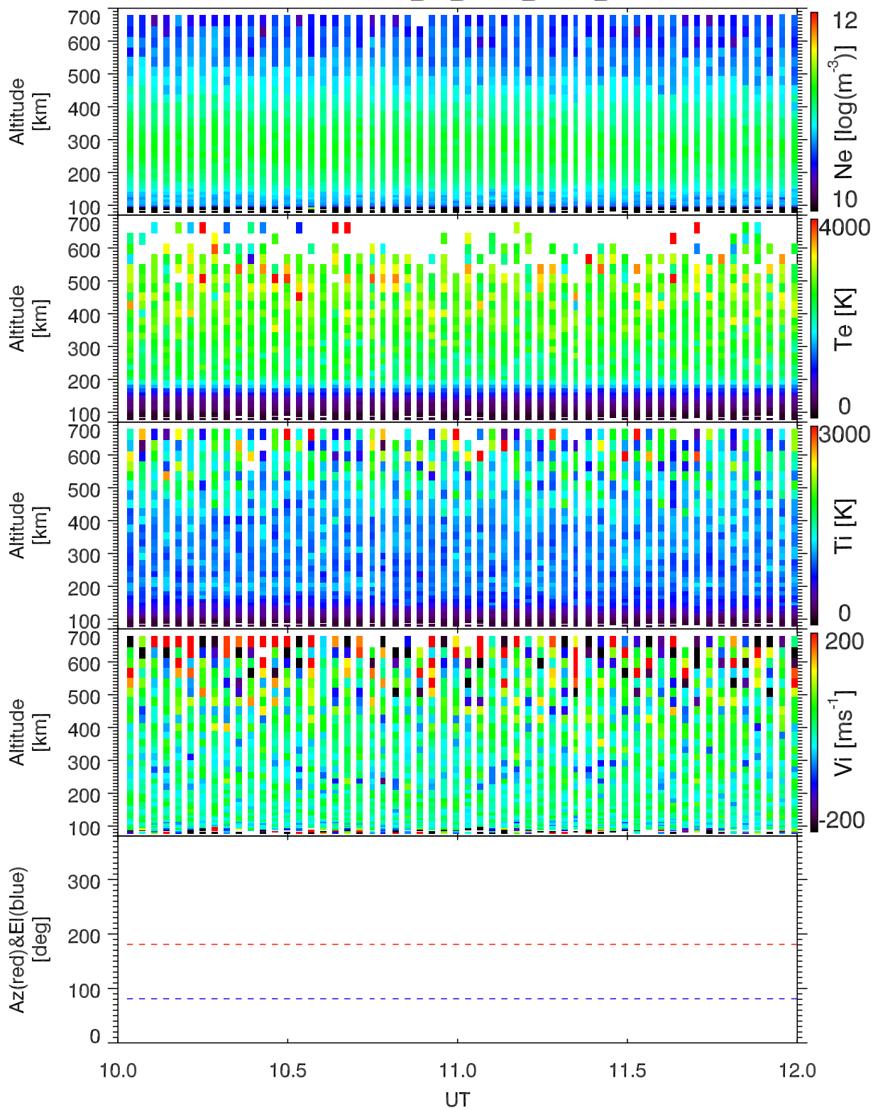
EISCAT 2004-06-10_10_12UT_steffe_ant@42m.
