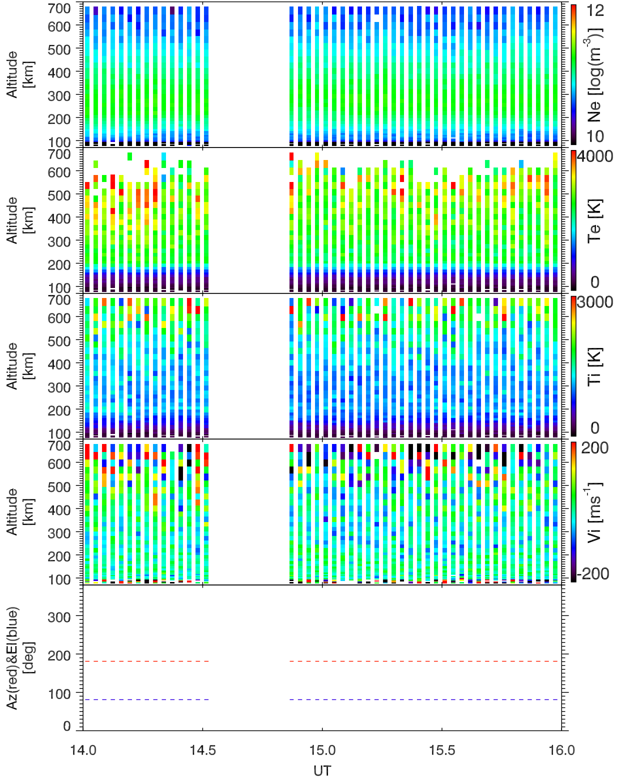
EISCAT 2004-06-10_14_16UT_steffe_ant@42m.
