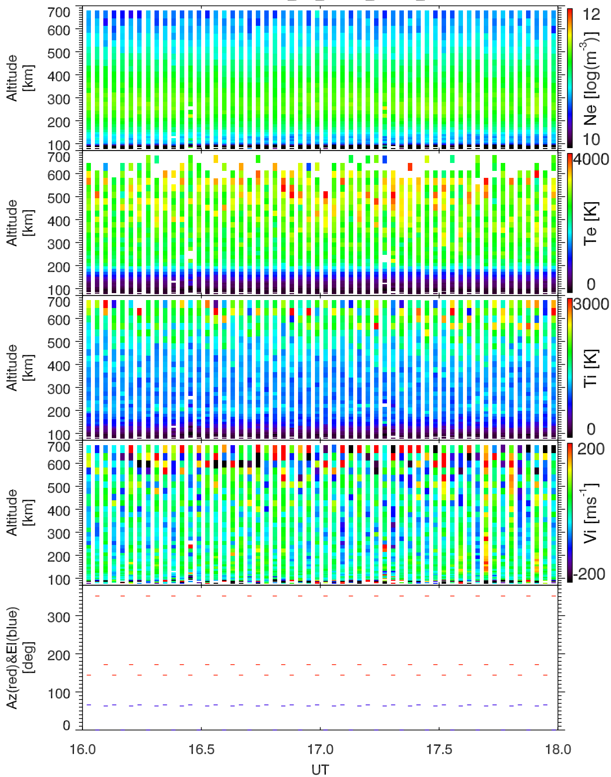
EISCAT 2004-06-10_16_18UT_steffe_ant@32m.
