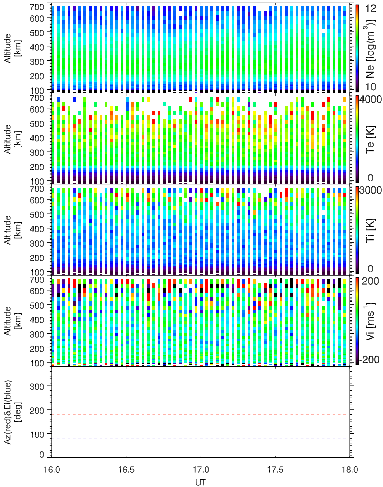
EISCAT 2004-06-10_16_18UT_steffe_ant@42m.
