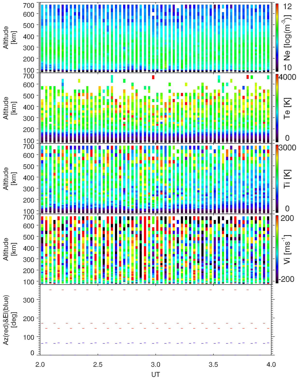
EISCAT 2004-06-11_02_04UT_steffe_ant@32m.
