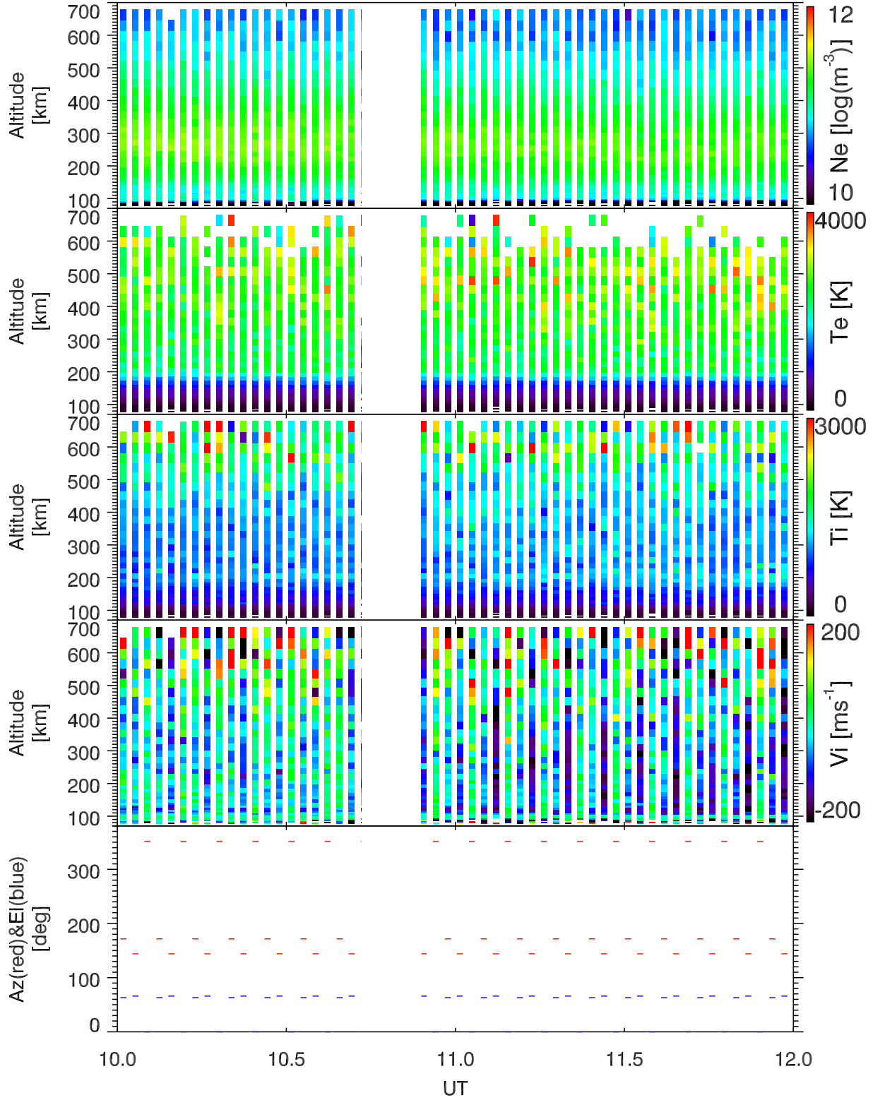
EISCAT 2004-06-11_10_12UT_steffe_ant@32m.
