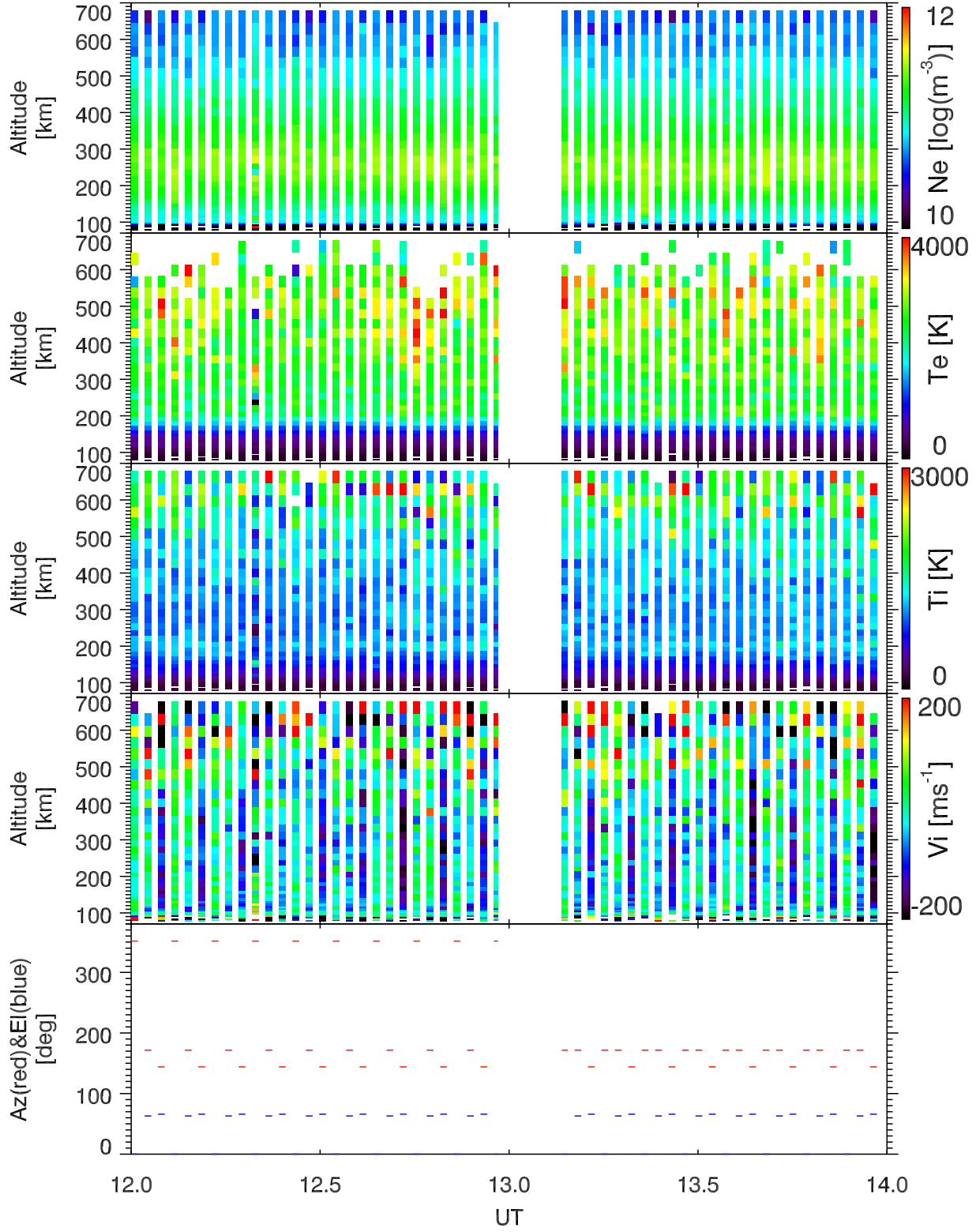
EISCAT 2004-06-11_12_14UT_steffe_ant@32m.
