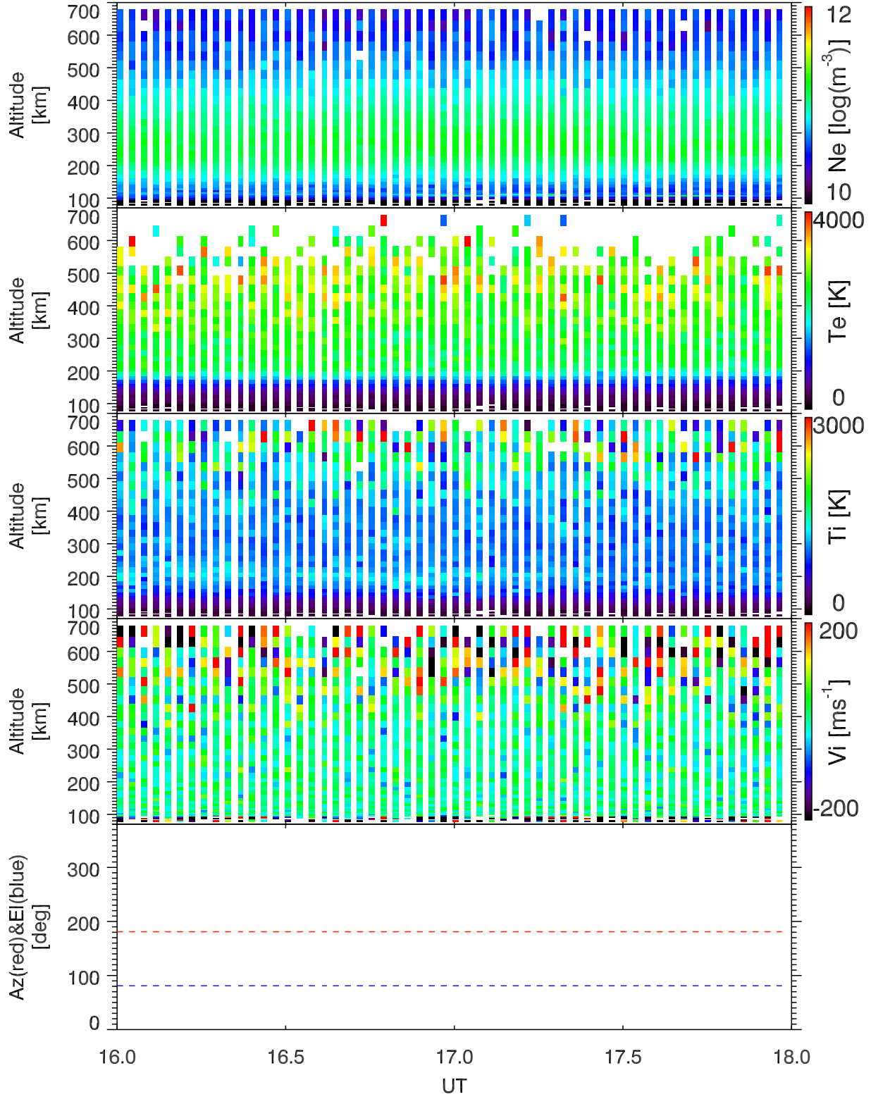
EISCAT 2004-06-11_16_18UT_steffe_ant@42m.
