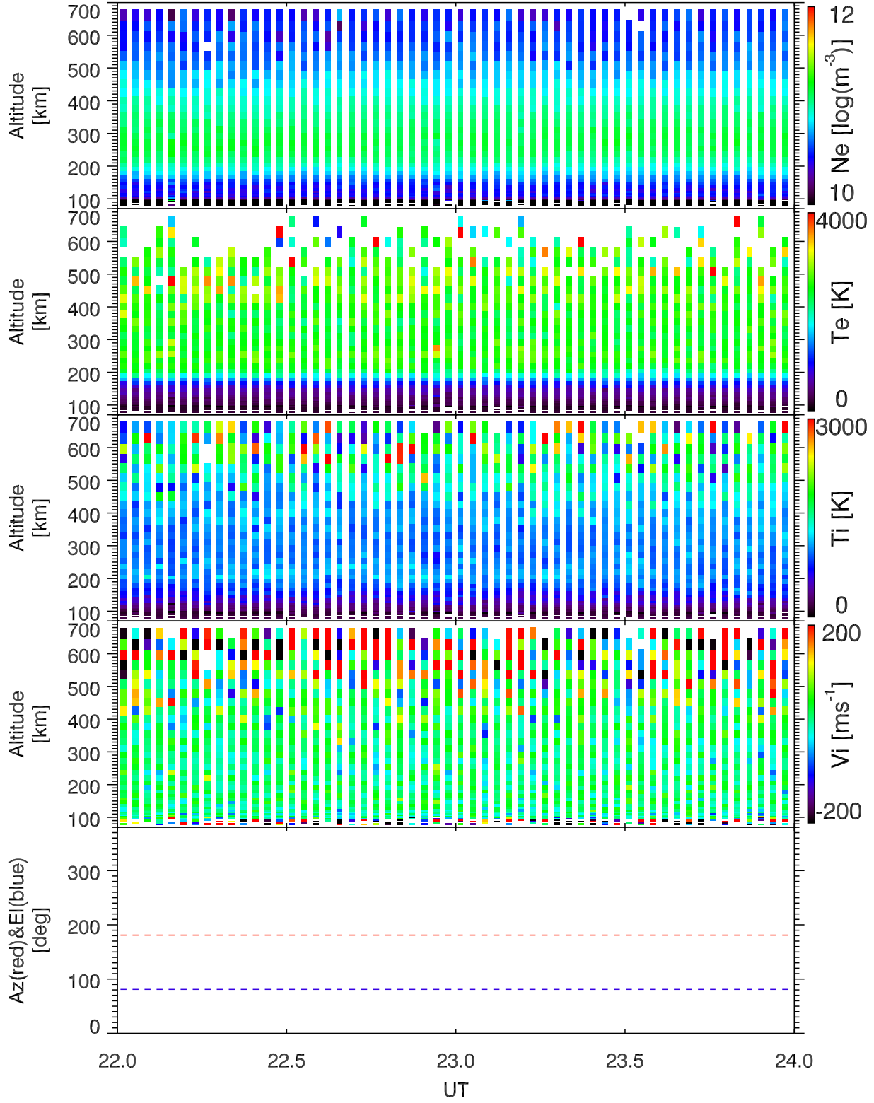
EISCAT 2004-06-11_22_24UT_steffe_ant@42m.
