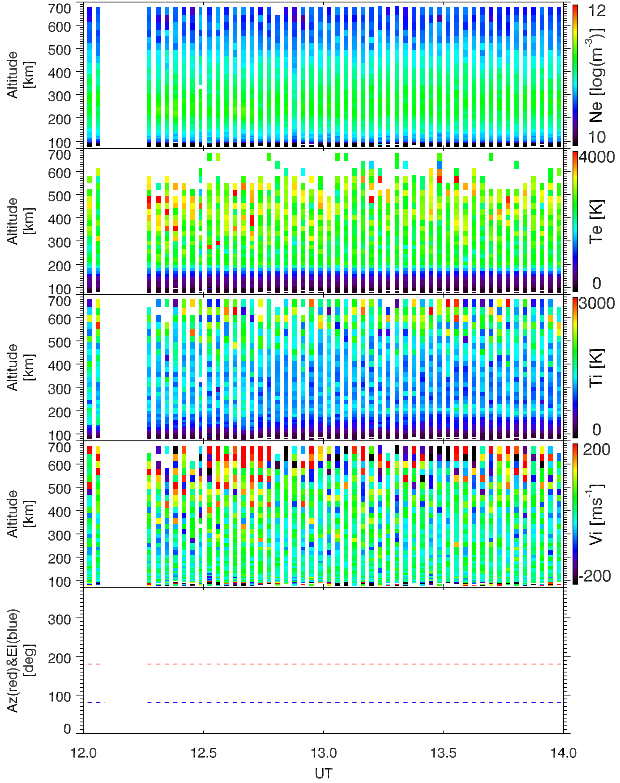
EISCAT 2004-06-12_12_14UT_steffe_ant@42m.
