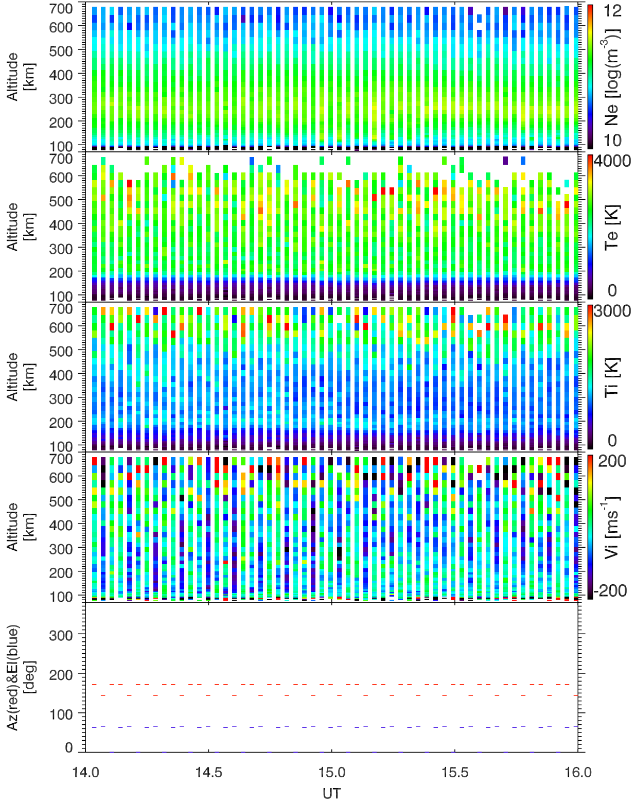
EISCAT 2004-06-12_14_16UT_steffe_ant@32m.
