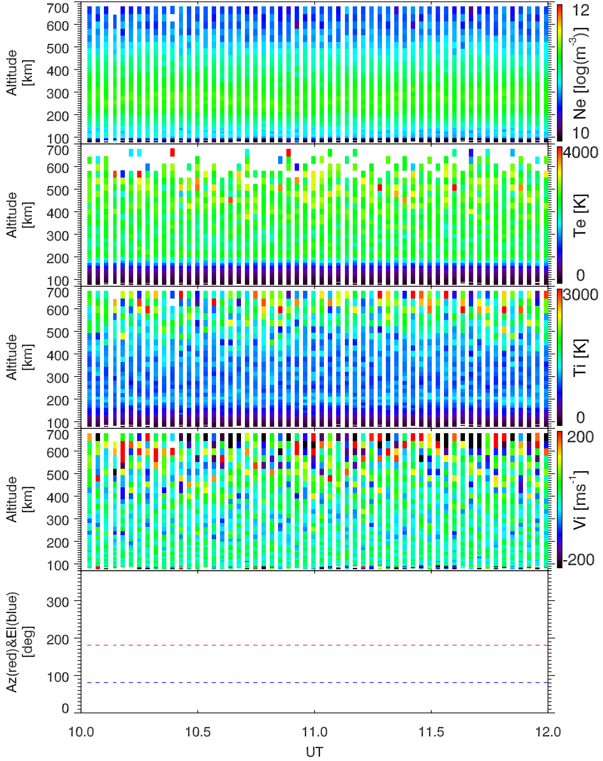
EISCAT 2004-06-13_10_12UT_steffe_ant@42m.
