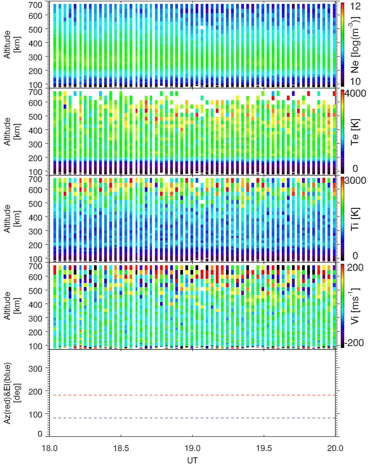
EISCAT 2004-06-13_18_20UT_steffe_ant@42m.
