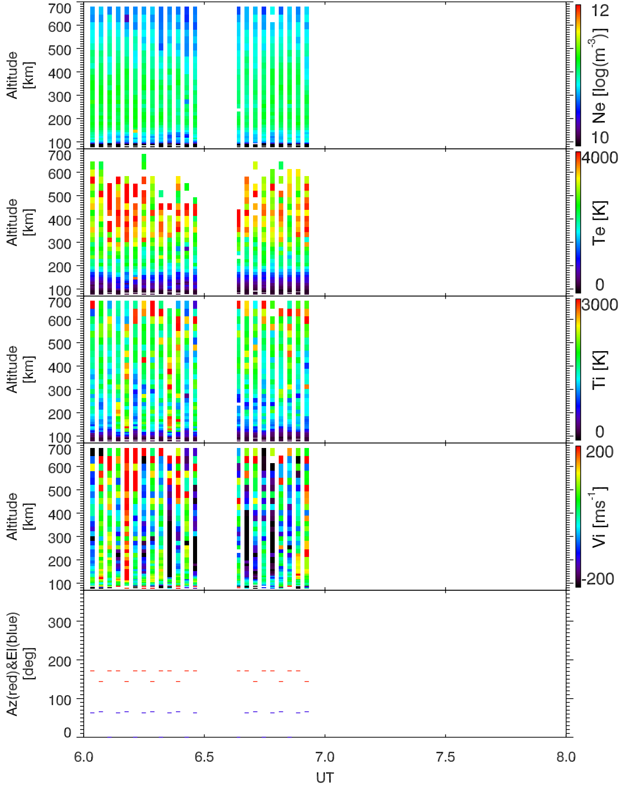
EISCAT 2004-06-14_06_08UT_steffe_ant@32m.
