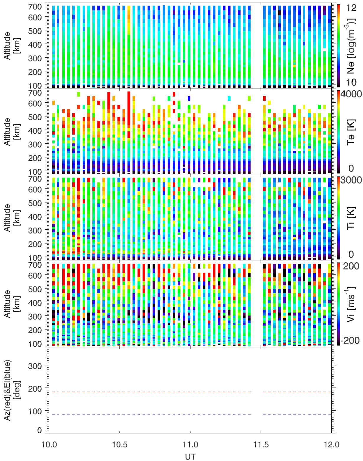
EISCAT 2005-06-13_10_12UT_steffe_ant@42m.
