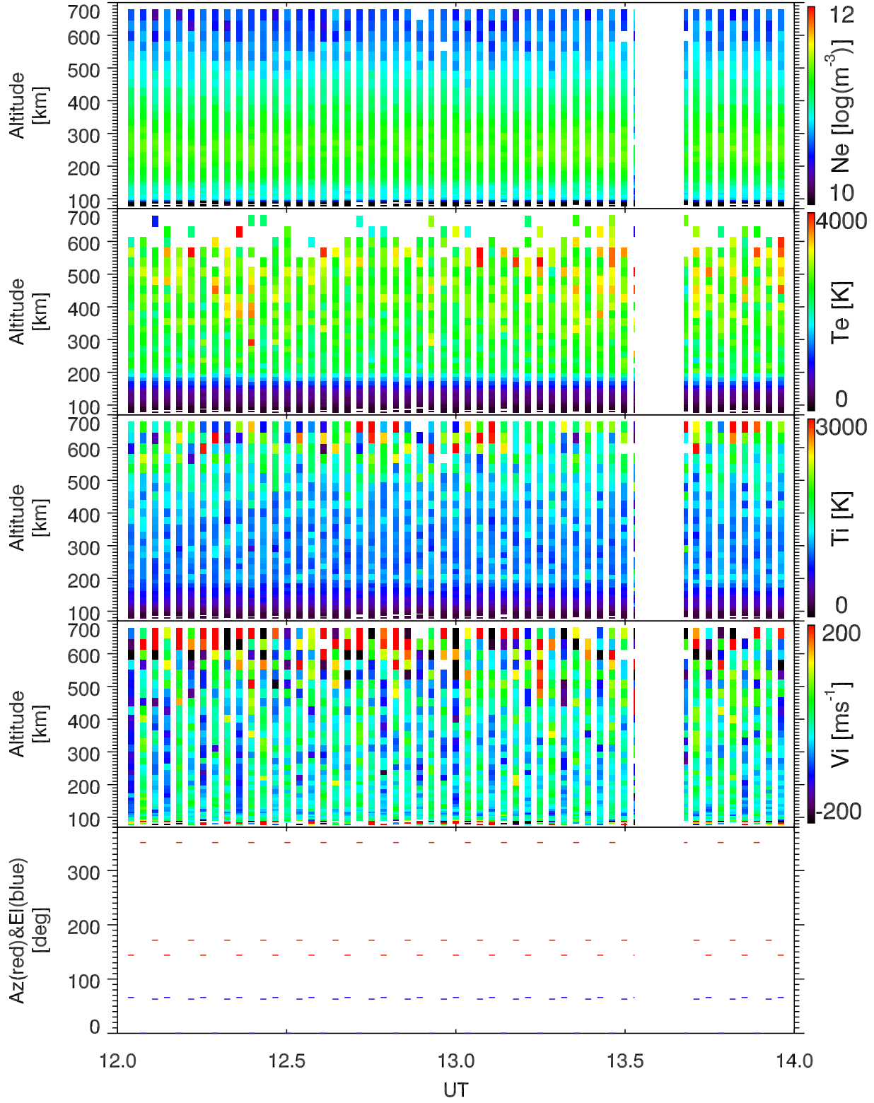
EISCAT 2005-06-14_12_14UT_steffe_ant@32m.
