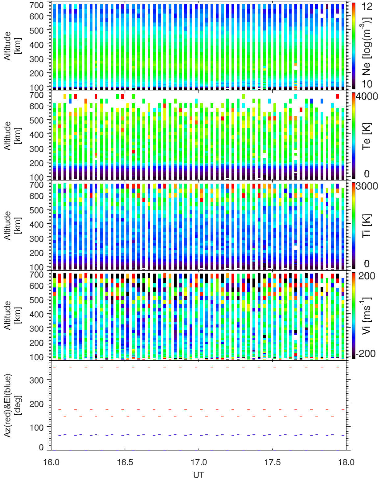
EISCAT 2005-06-14_16_18UT_steffe_ant@32m.
