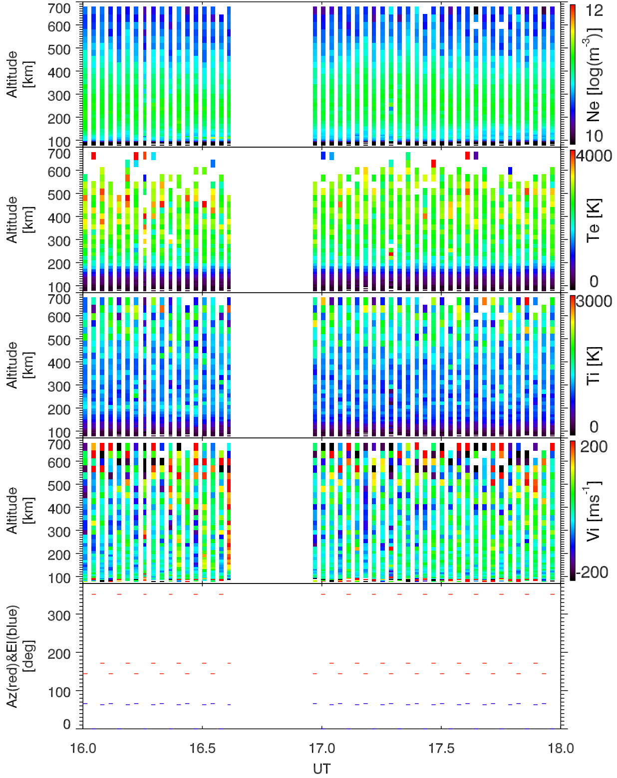
EISCAT 2005-06-15_16_18UT_steffe_ant@32m.
