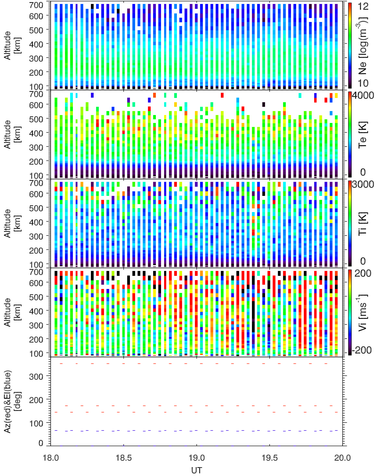
EISCAT 2005-06-16_18_20UT_steffe_ant@32m.
