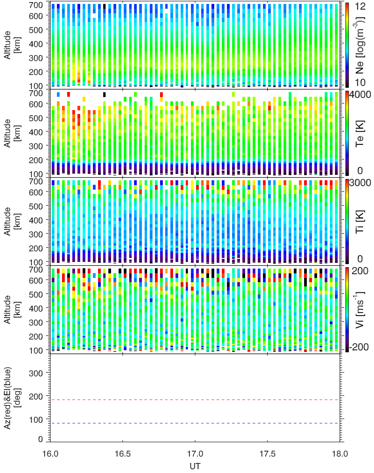
EISCAT 2005-07-01_16_18UT_tau0_ant@42m.
