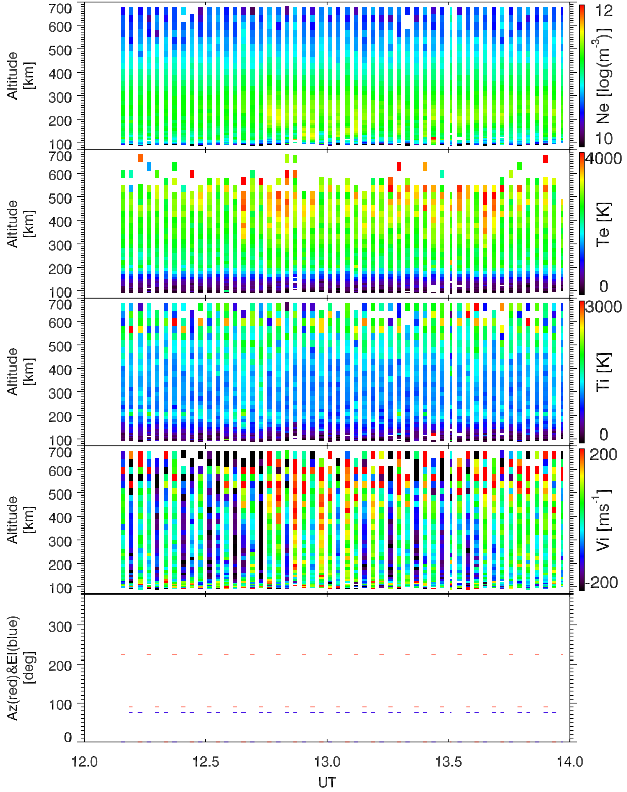
EISCAT 2005-07-22_12_14UT_tau0_ant@32m.
