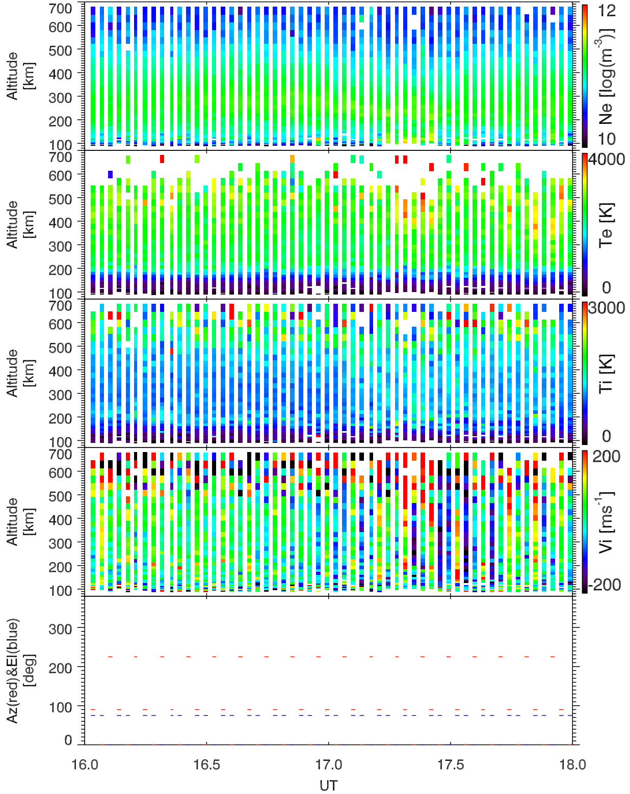
EISCAT 2005-07-22_16_18UT_tau0_ant@32m.
