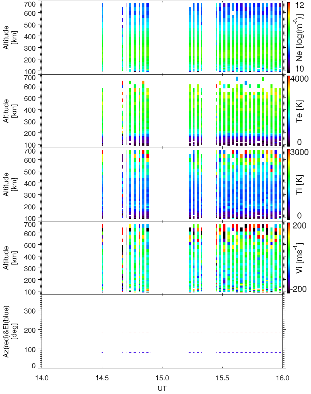
EISCAT 2005-07-23_14_16UT_tau0_ant@42m.
