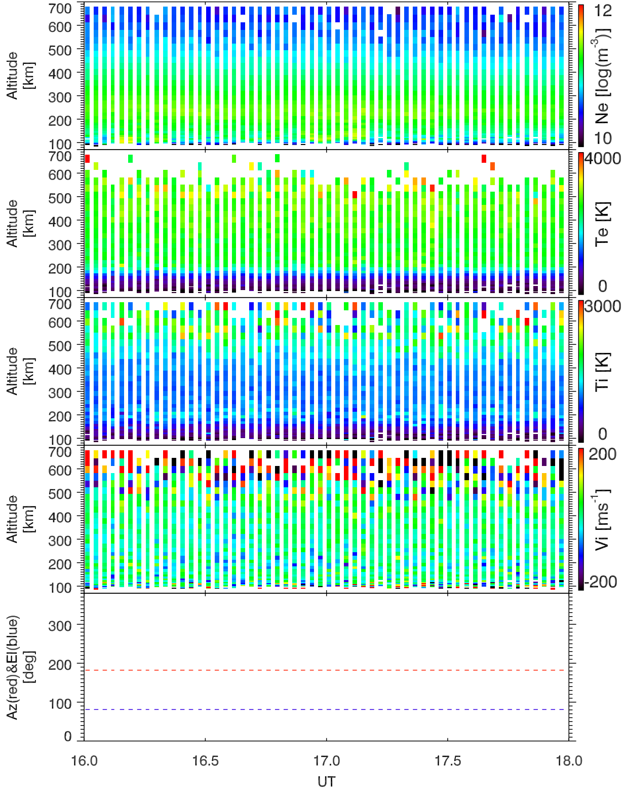
EISCAT 2005-07-23_16_18UT_tau0_ant@42m.
