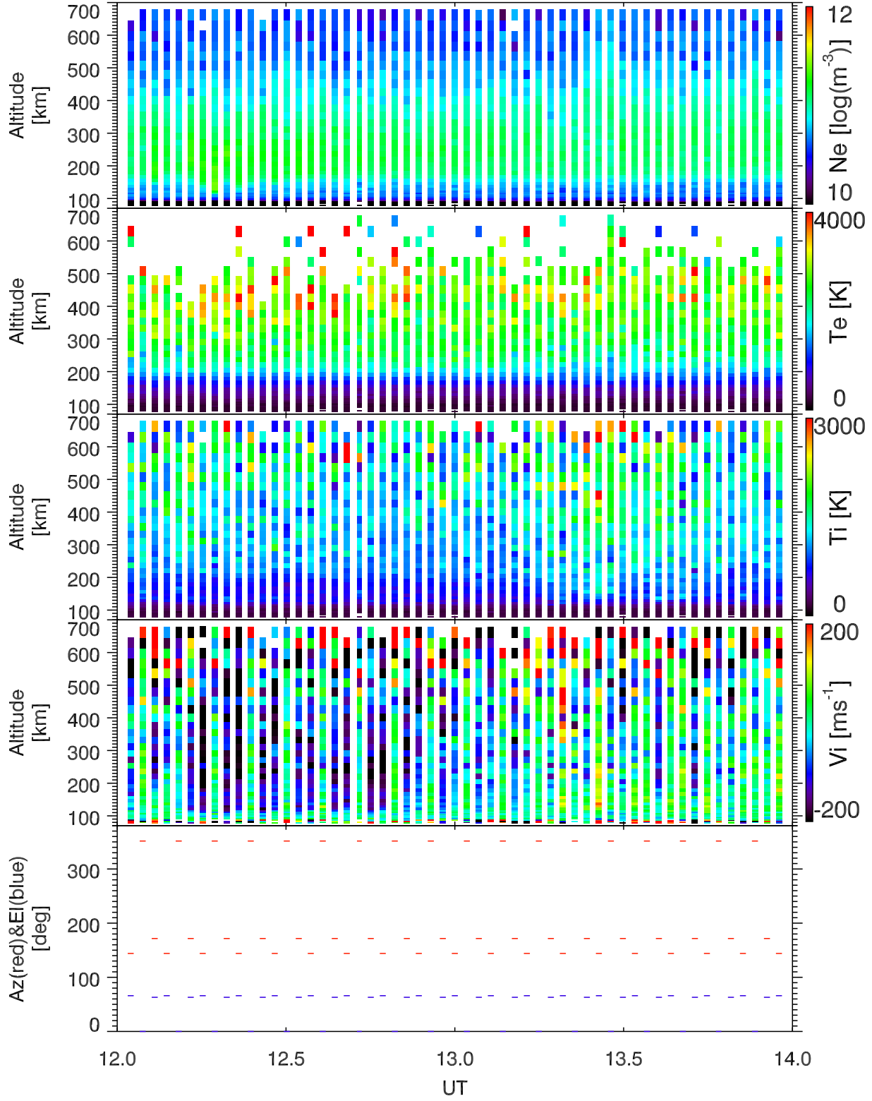
EISCAT 2005-09-03_12_14UT_steffe_ant@32m.
