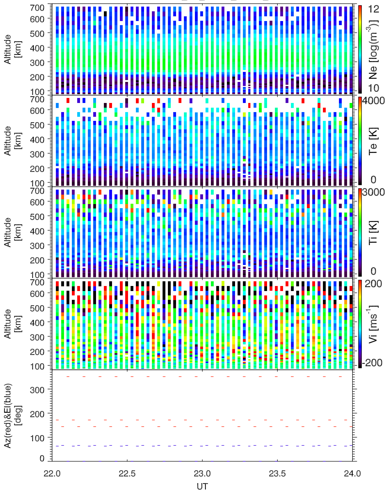
EISCAT 2005-09-09_22_24UT_steffe_ant@32m.
