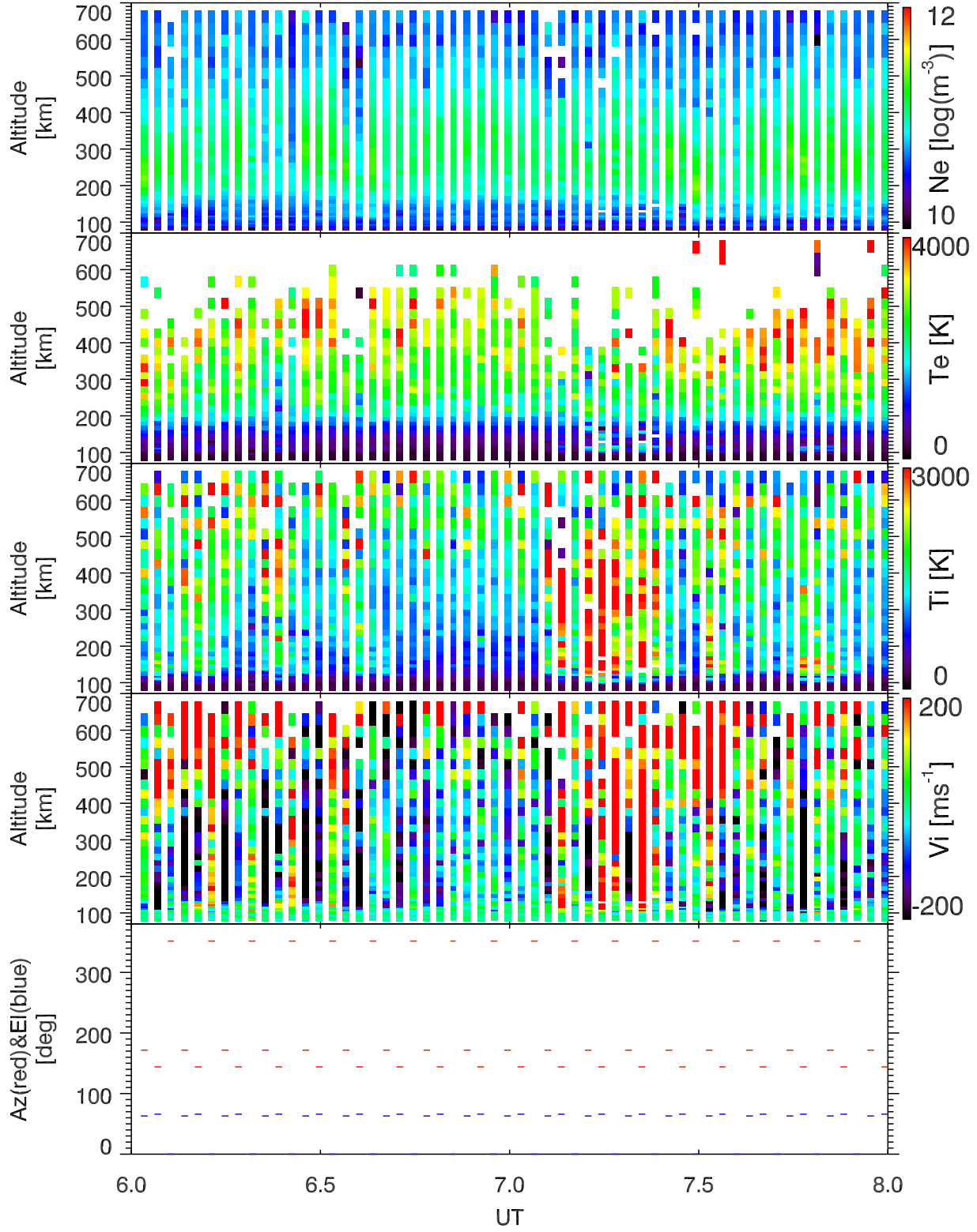
EISCAT 2005-09-10_06_08UT_steffe_ant@32m.
