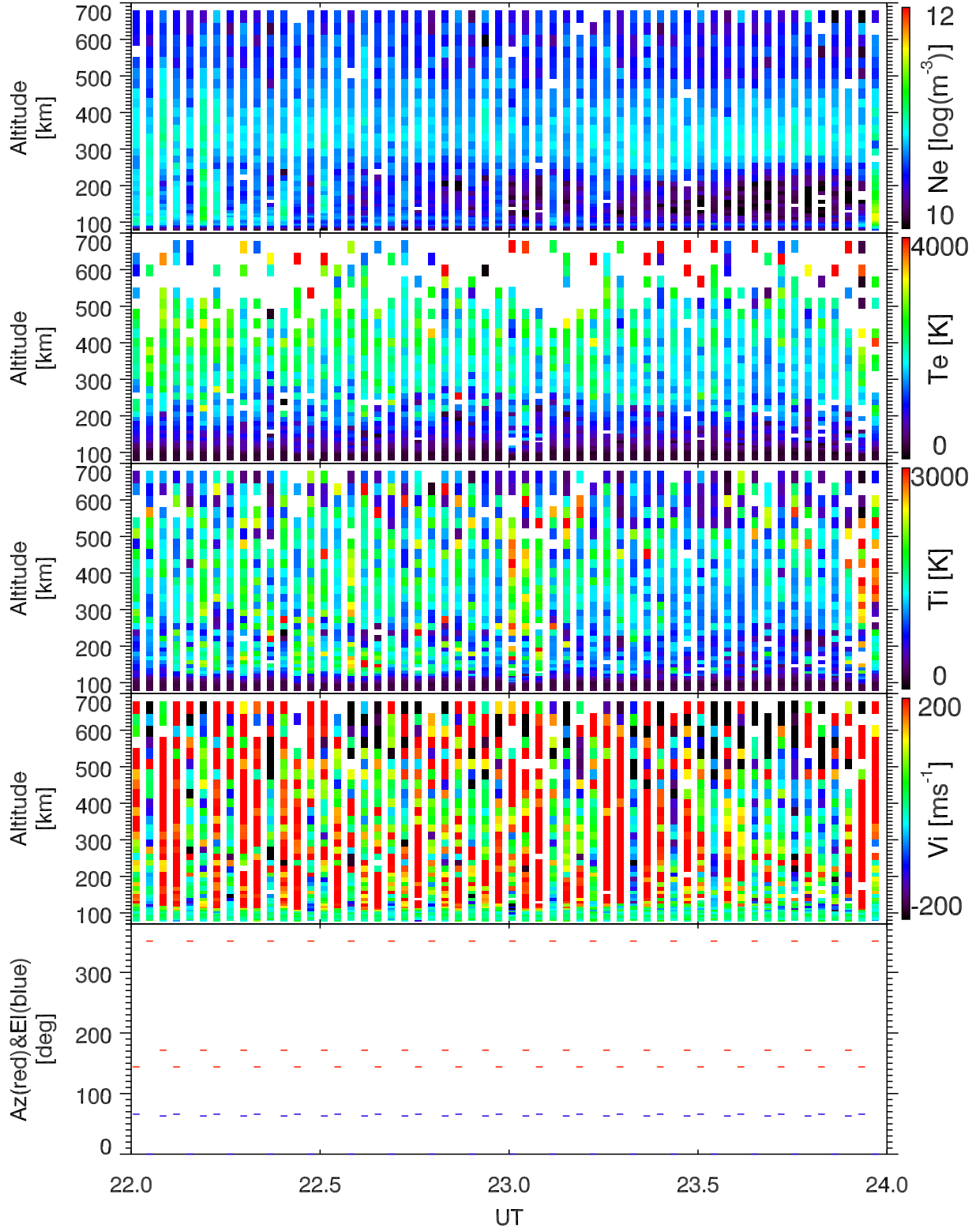
EISCAT 2005-09-11_22_24UT_steffe_ant@32m.
