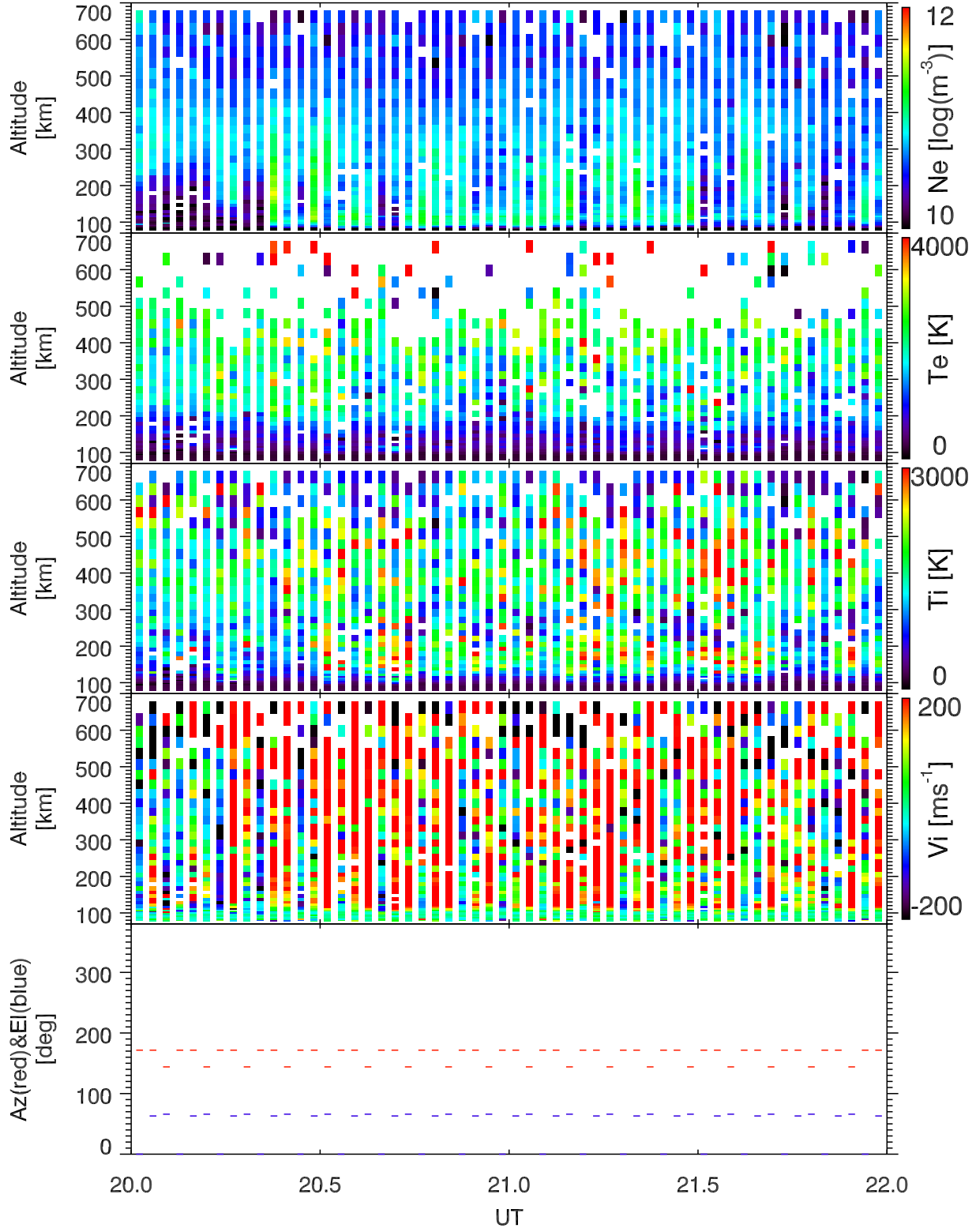
EISCAT 2005-09-15_20_22UT_steffe_ant@32m.
