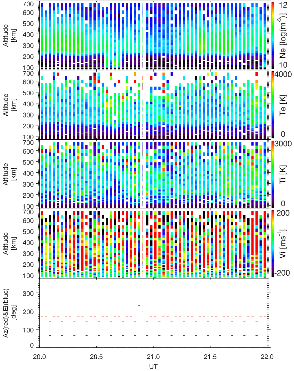
EISCAT 2005-09-16_20_22UT_steffe_ant@32m.
