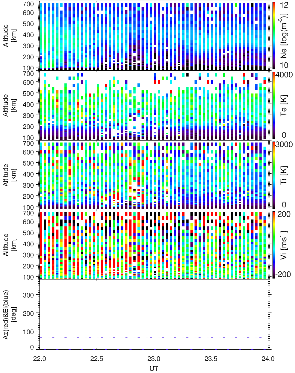
EISCAT 2005-09-16_22_24UT_steffe_ant@32m.
