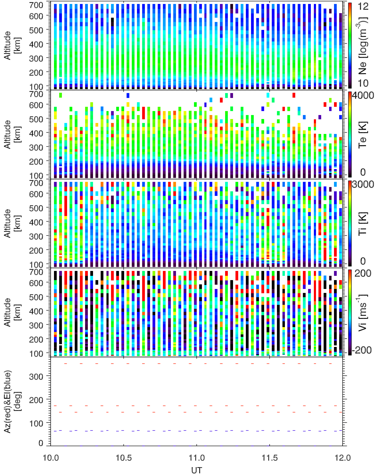
EISCAT 2005-09-17_10_12UT_steffe_ant@32m.
