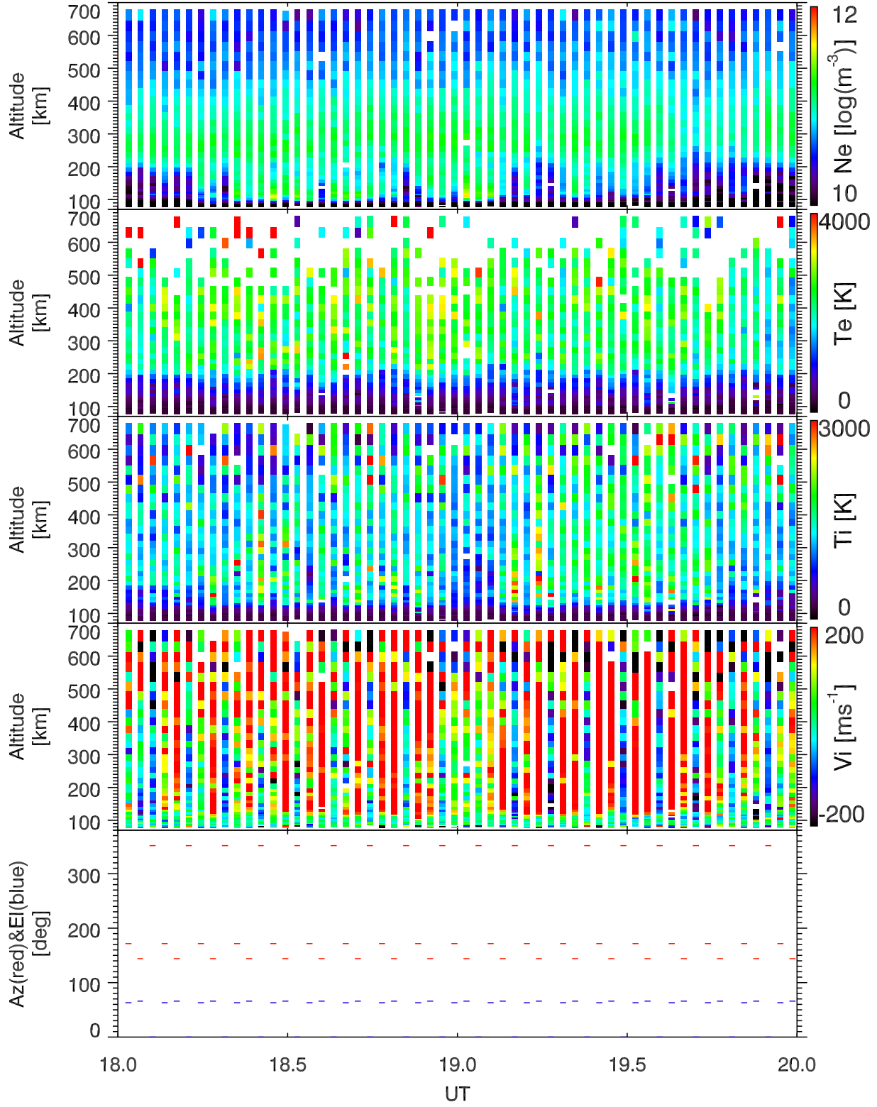
EISCAT 2005-09-18_18_20UT_steffe_ant@32m.
