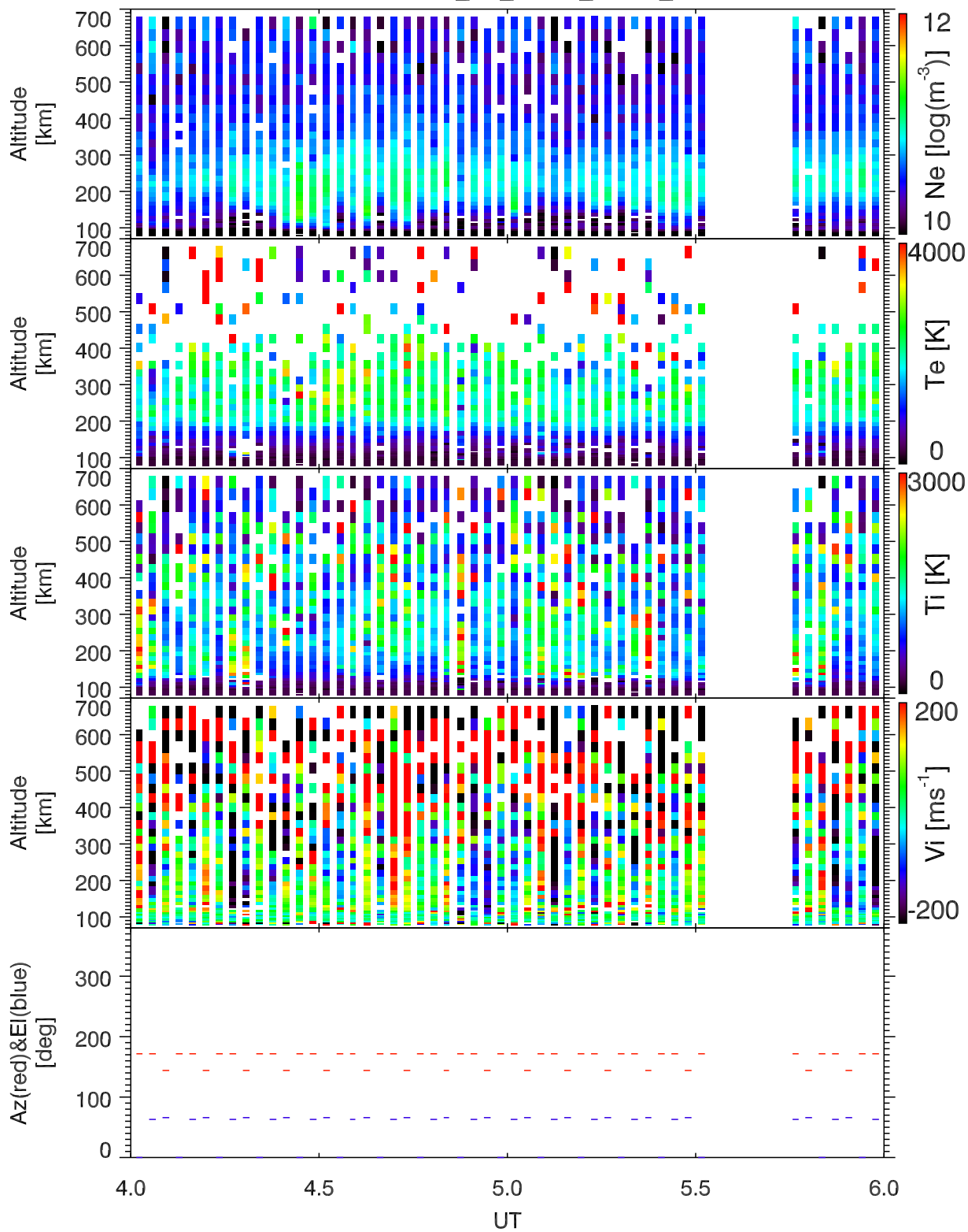
EISCAT 2005-09-20_04_06UT_steffe_ant@32m.
