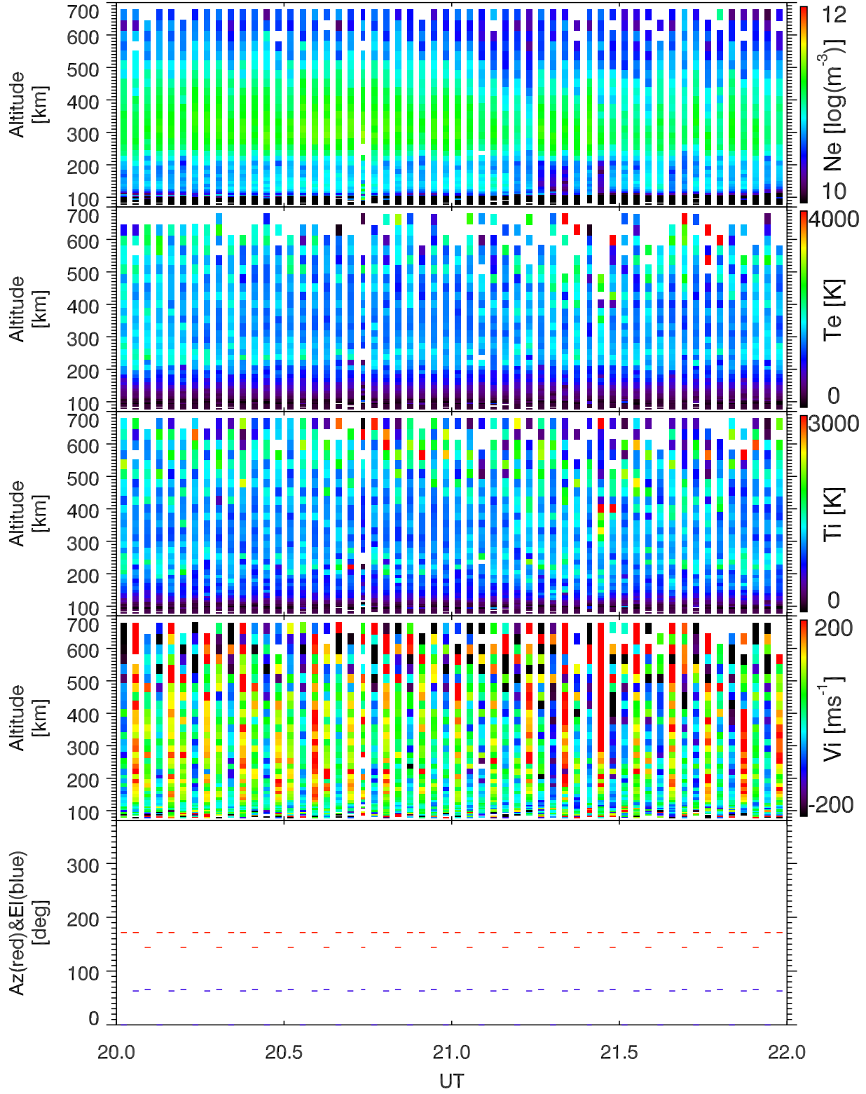
EISCAT 2005-09-20_20_22UT_steffe_ant@32m.
