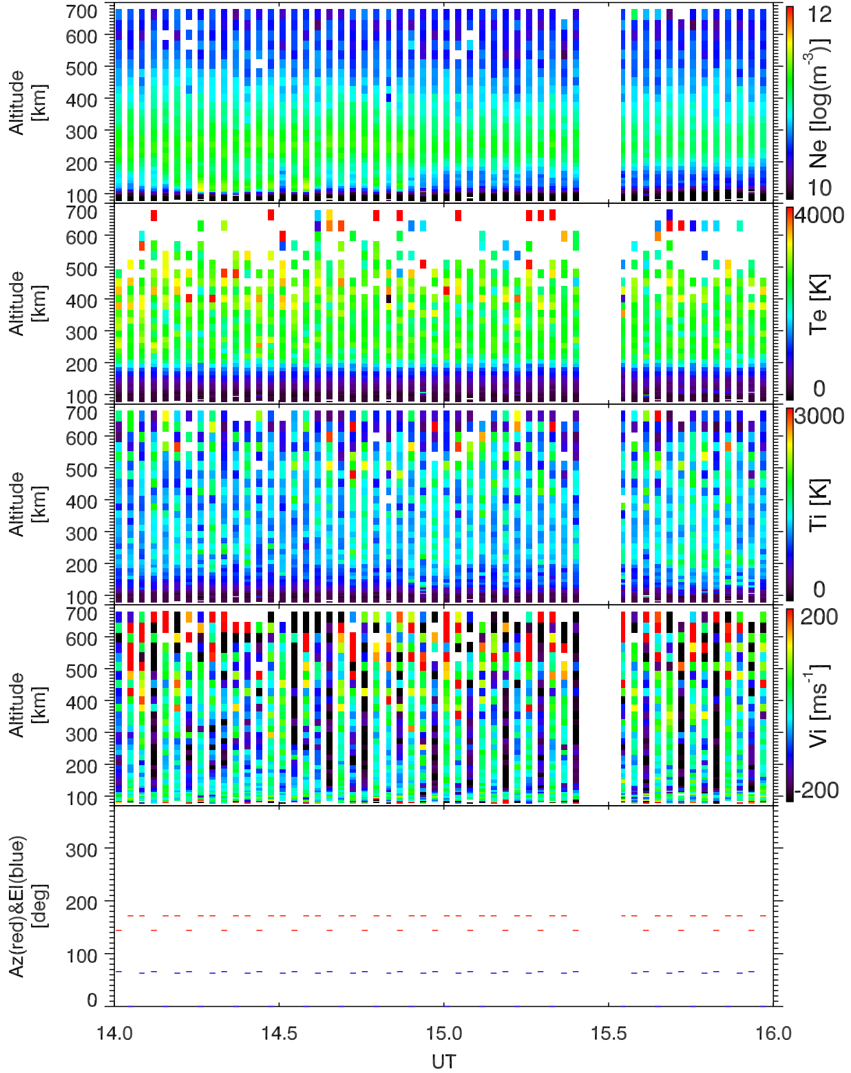
EISCAT 2005-09-21_14_16UT_steffe_ant@32m.
