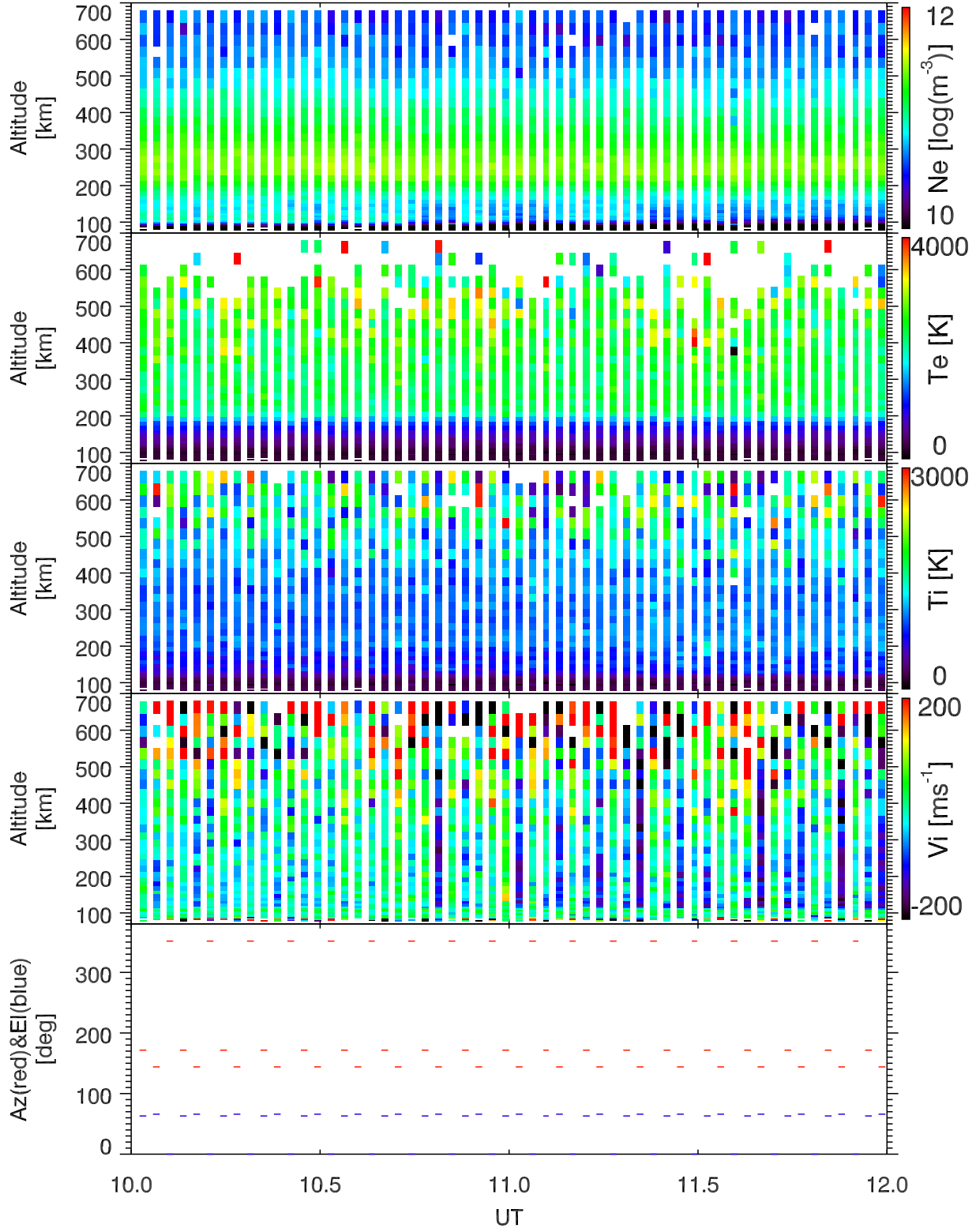
EISCAT 2005-09-24_10_12UT_steffe_ant@32m.
