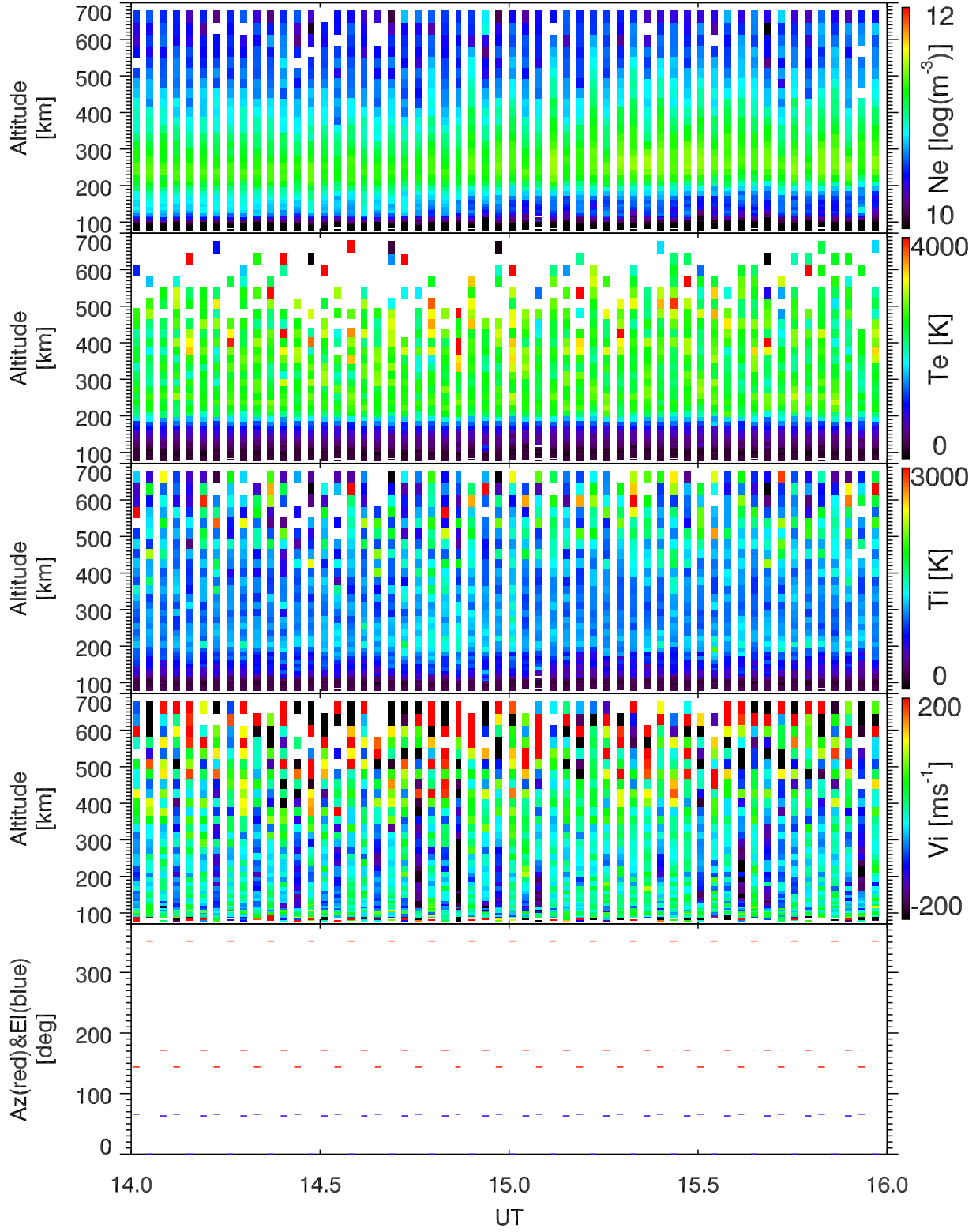
EISCAT 2005-09-24_14_16UT_steffe_ant@32m.
