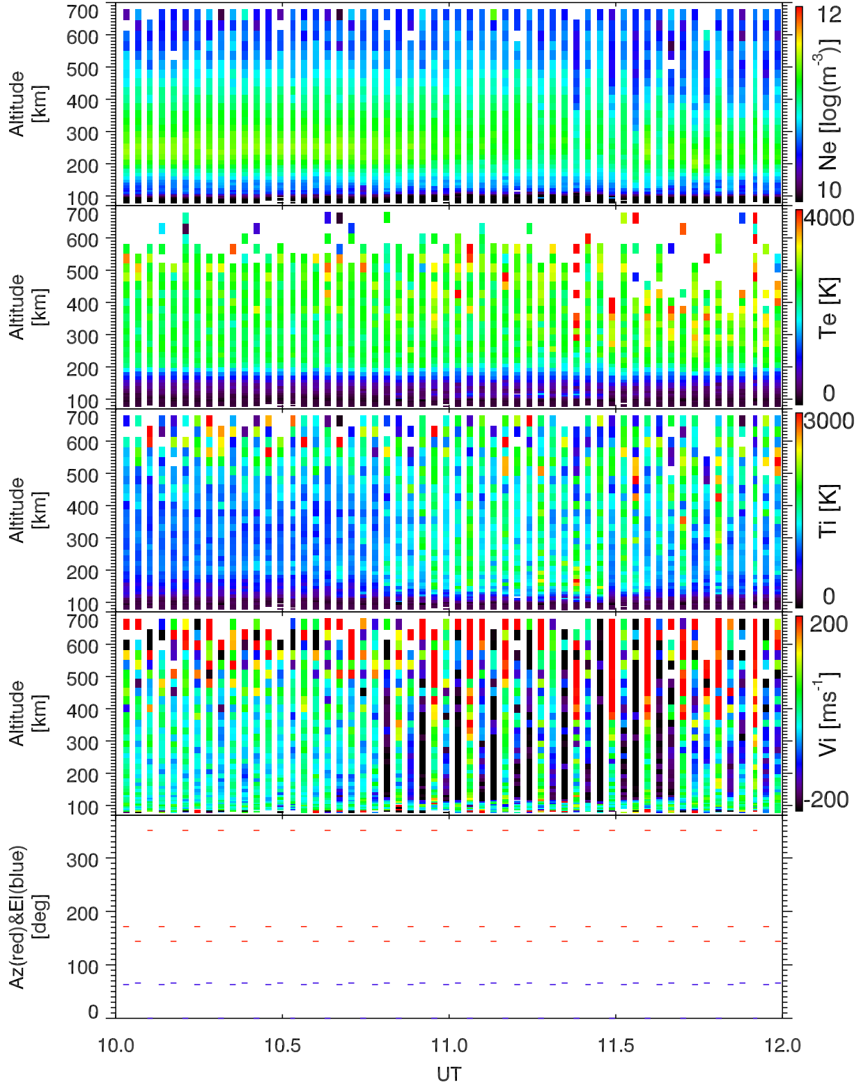
EISCAT 2005-09-25_10_12UT_steffe_ant@32m.
