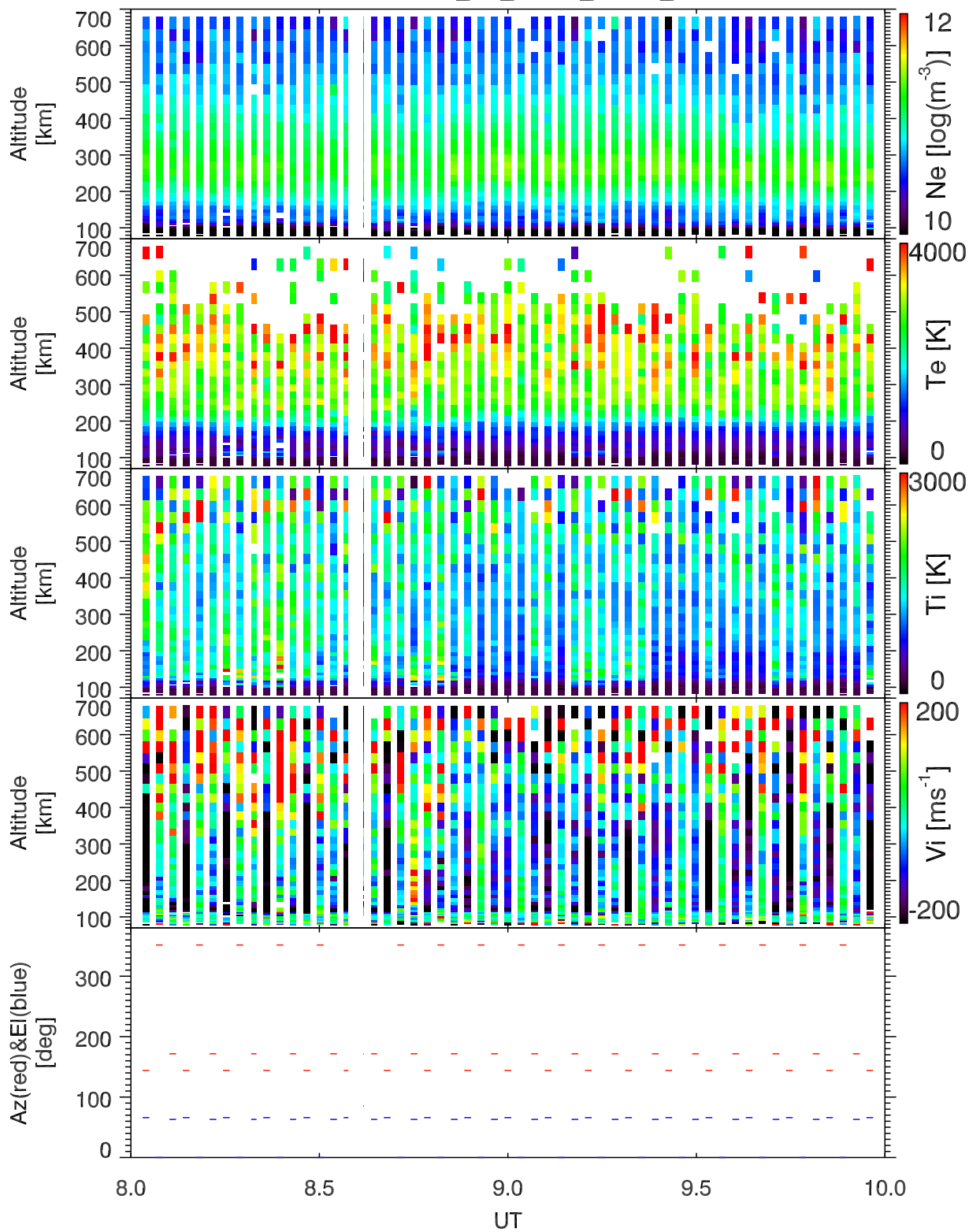
EISCAT 2005-09-27_08_10UT_steffe_ant@32m.
