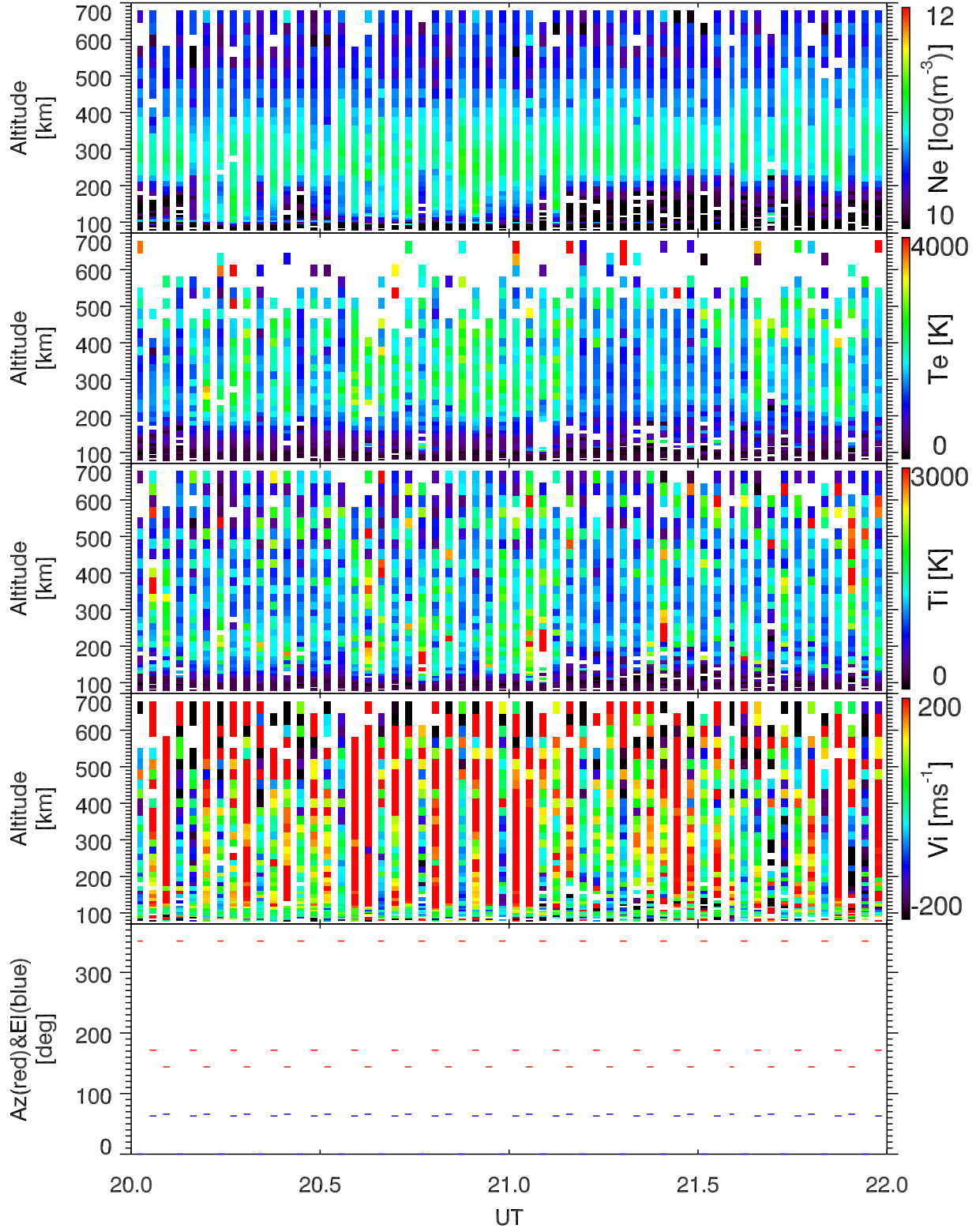
EISCAT 2005-09-27_20_22UT_steffe_ant@32m.
