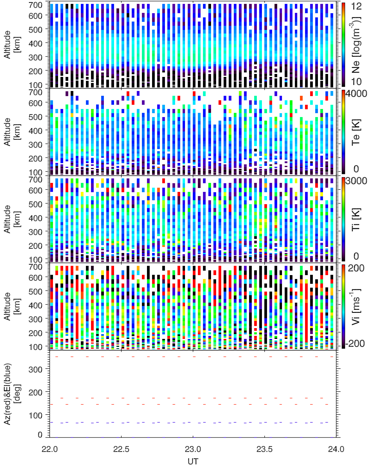
EISCAT 2005-09-27_22_24UT_steffe_ant@32m.
