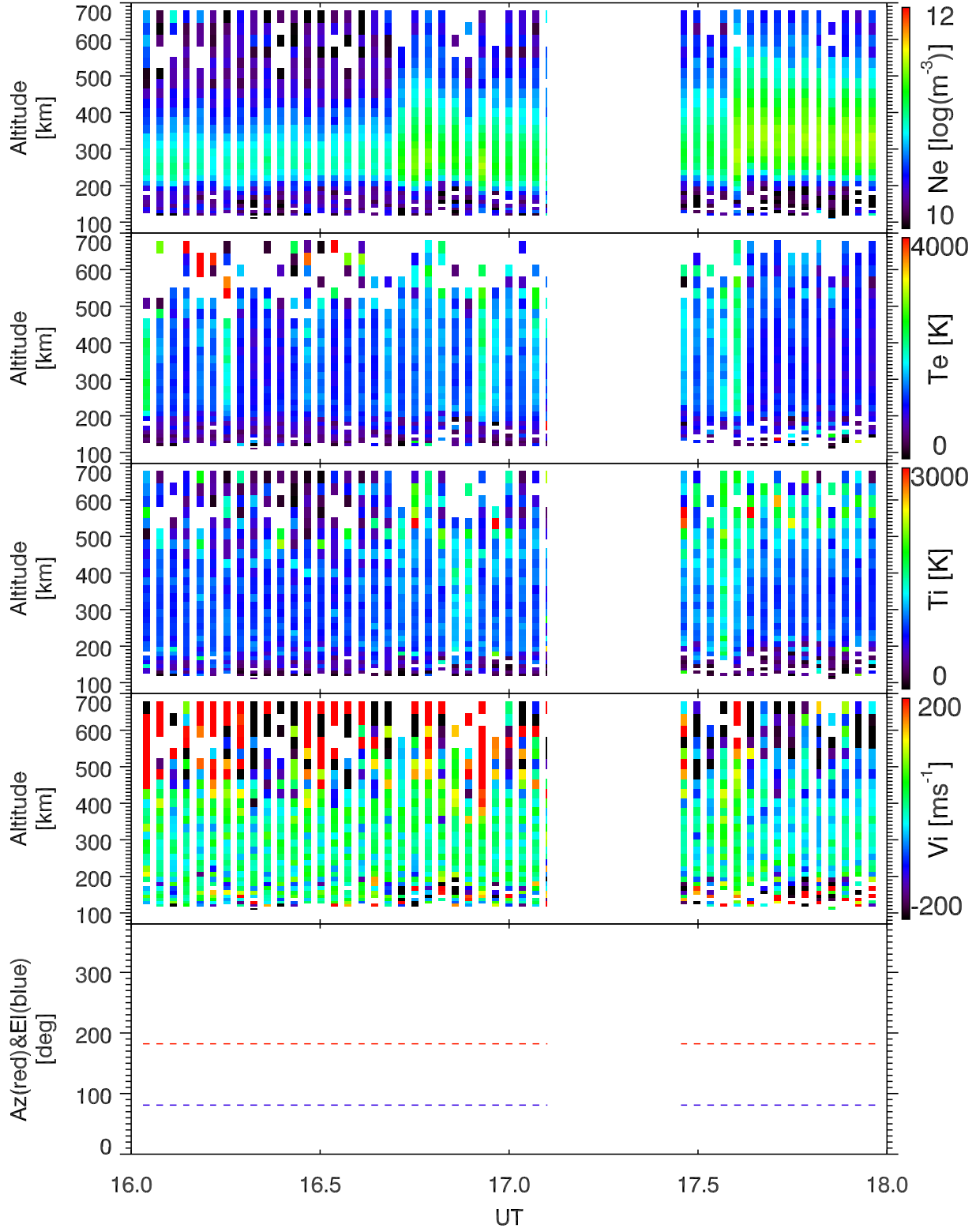
EISCAT 2005-11-10_16_18UT_tau0_ant@42m.
