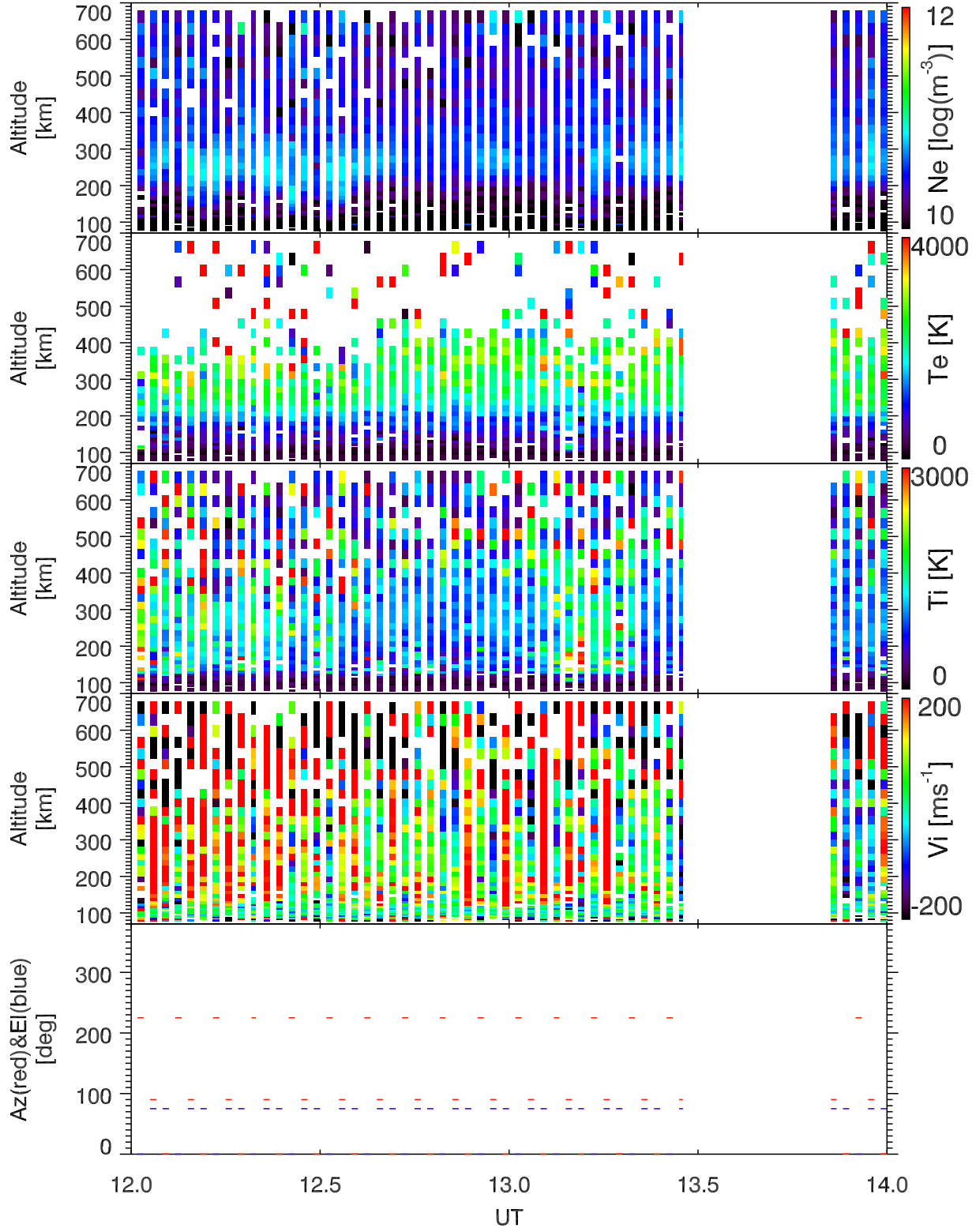
EISCAT 2006-02-21_12_14UT_steffe_ant@32m.
