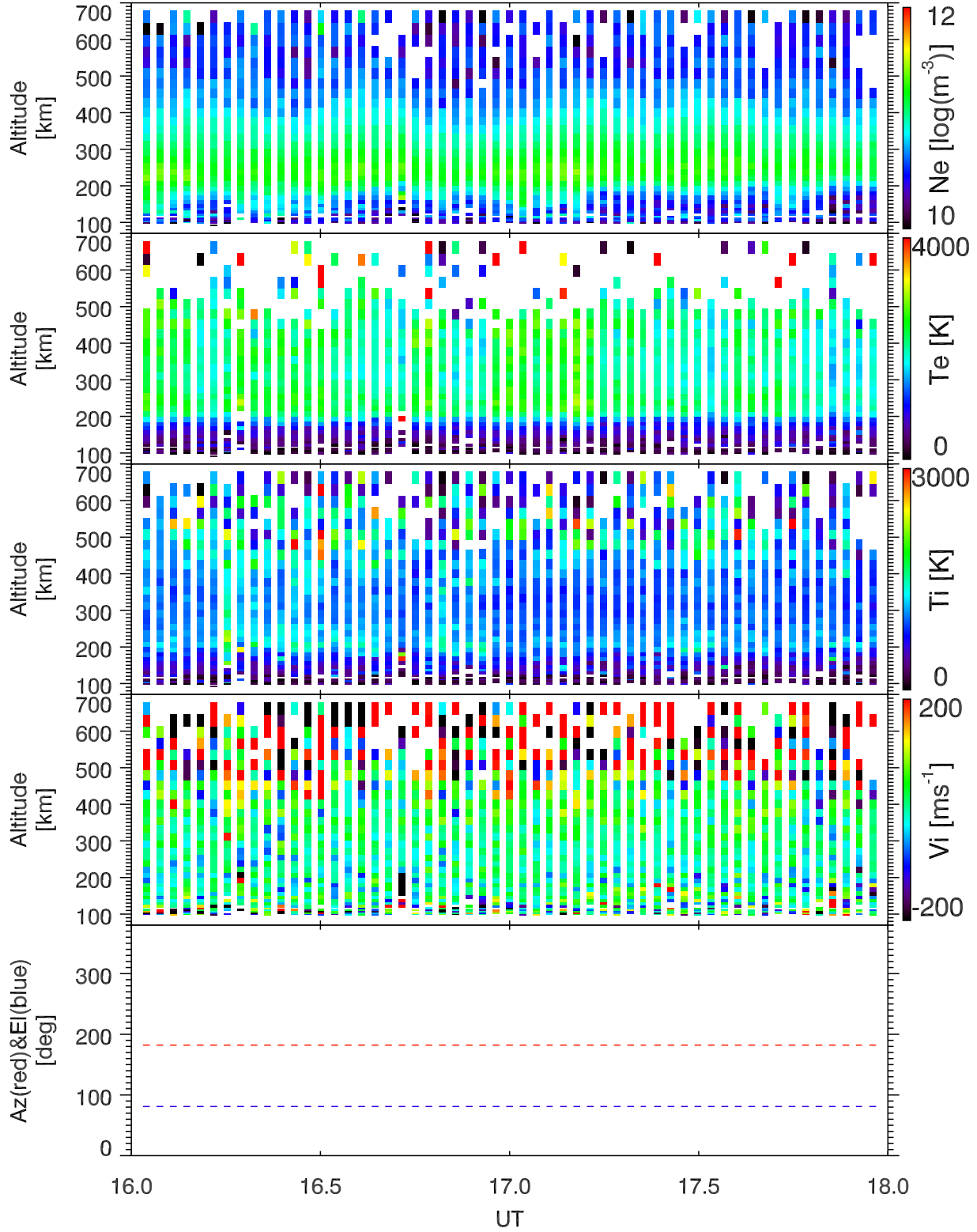
EISCAT 2006-09-20_16_18UT_tau0_ant@42m.
