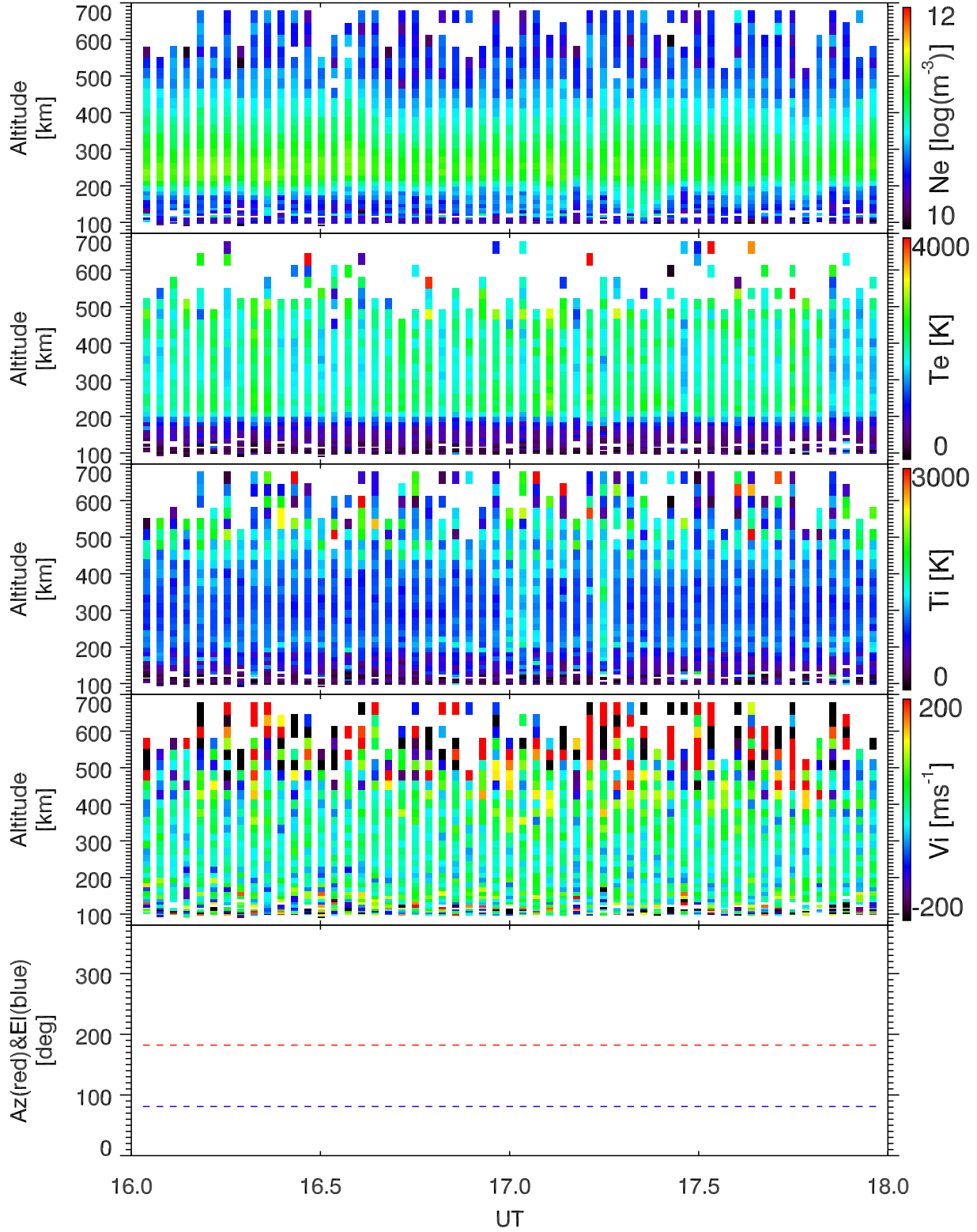
EISCAT 2006-09-21_16_18UT_tau0_ant@42m.
